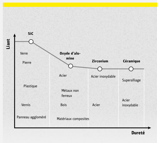
Classification du grain par rapport au liant, à la dureté et aux applications principales
